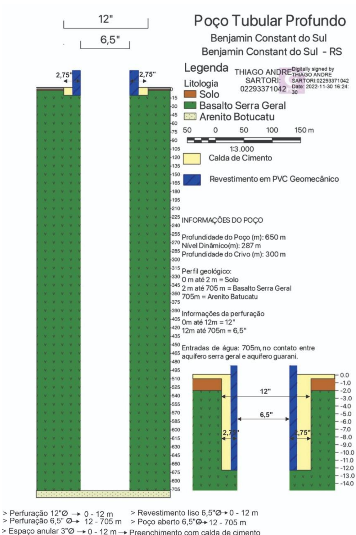
Fig 3: Perfil Hidrogeológico Construtivo feito pela empresa perfuradora
