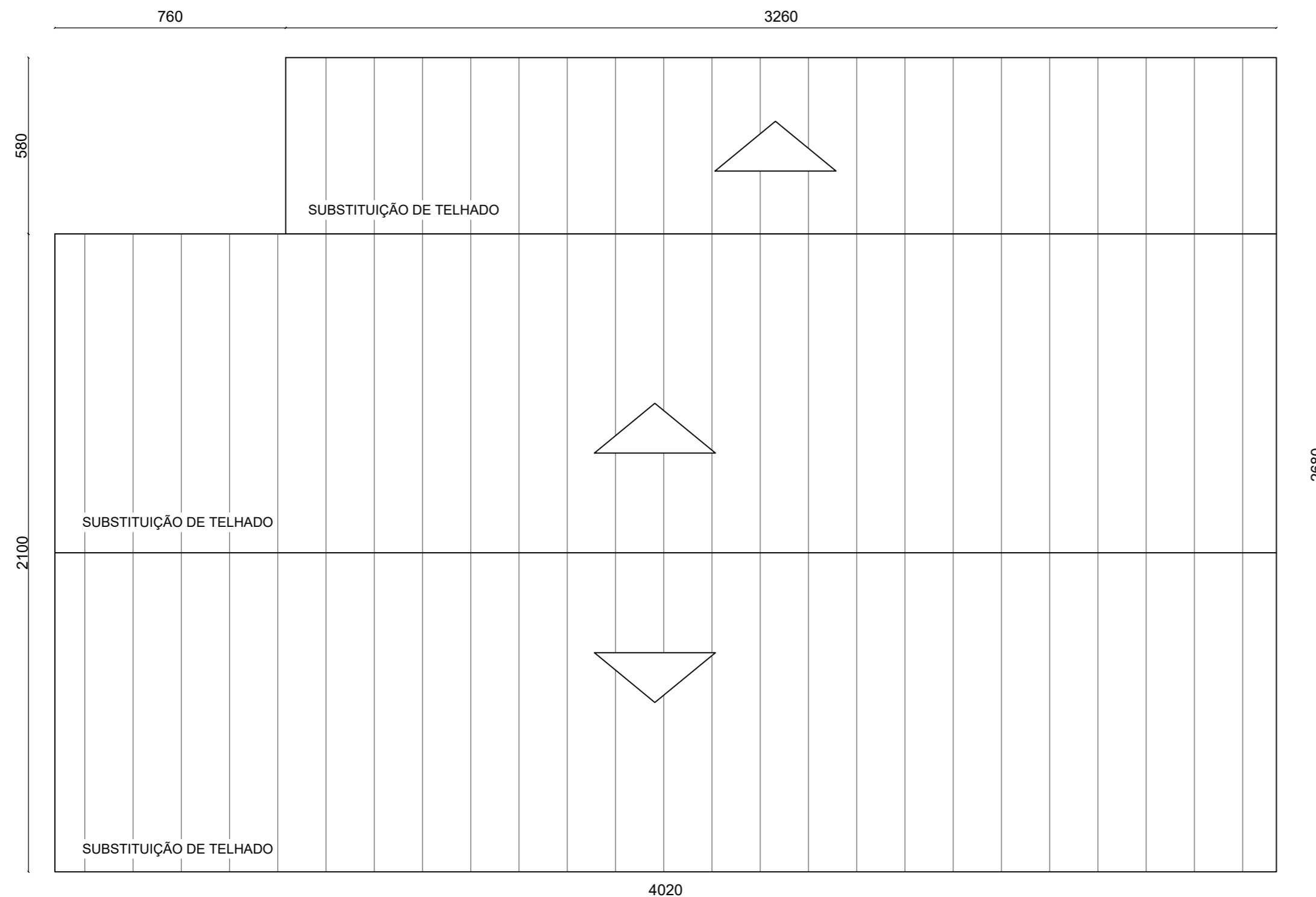
PLANTA BAIXA TELHADO GINÁSIO DE ESPORTES ESCALA 1:150
